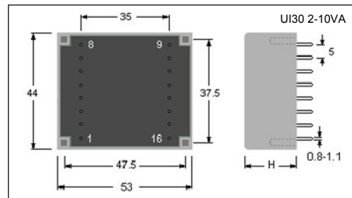
Dimensioni fisiche in mm Physical dimensions in mm
